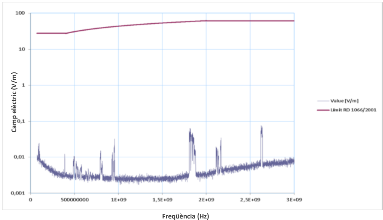
Figura 4. Valors de camp elèctric obtinguts per les freqüències entre 75 MHz i 3 GHz al punt 4.
