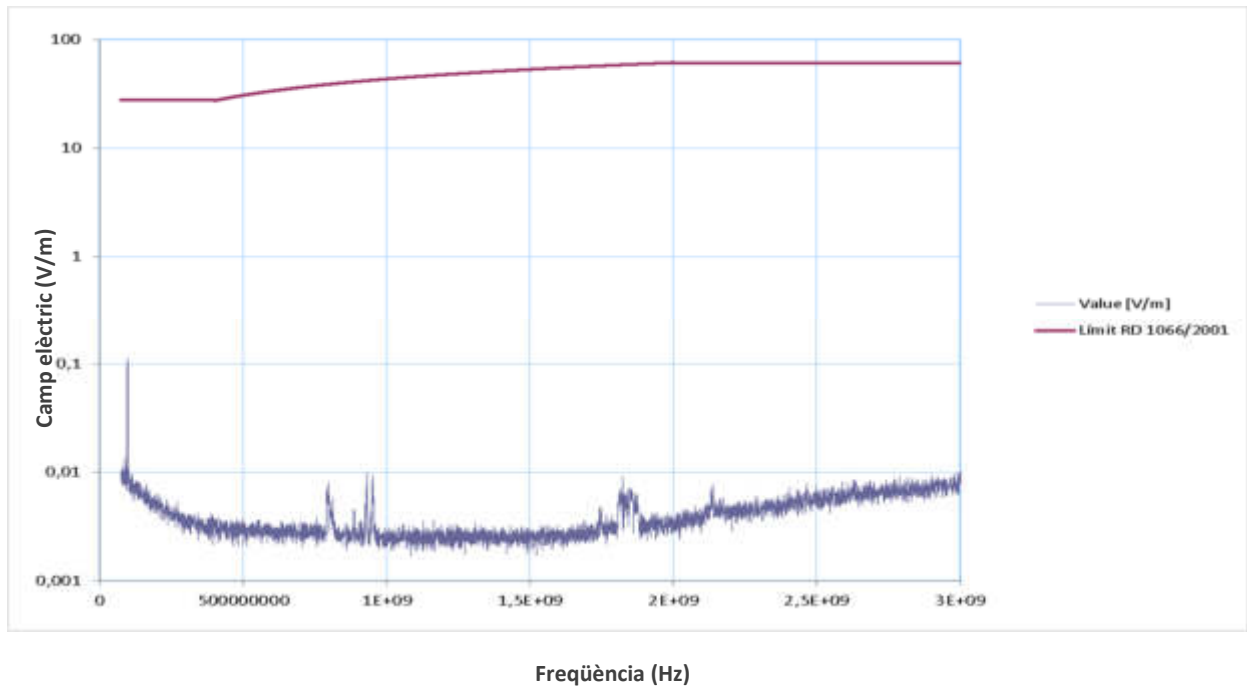
Figura 8. Valors de camp elèctric obtinguts per les freqüències entre 75 MHz i 3 GHz al punt 8.
