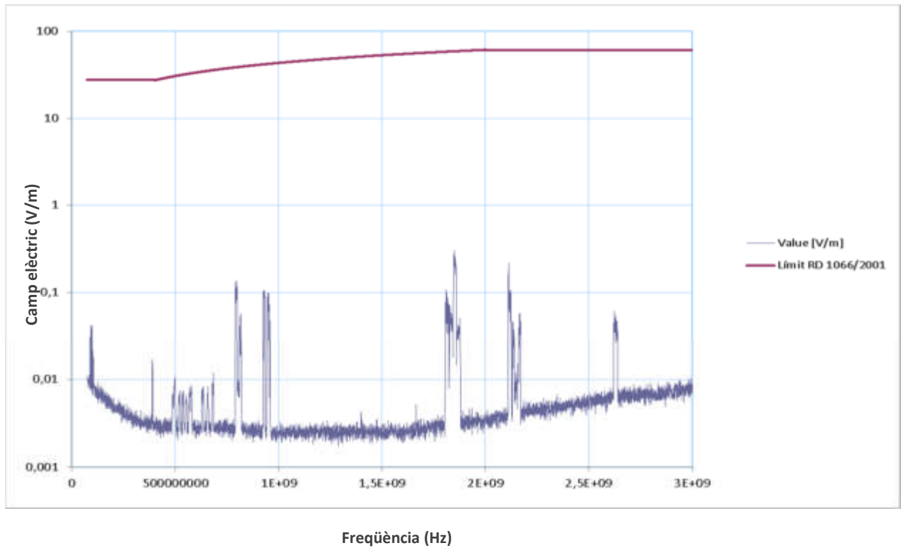
Figura 9. Valors de camp elèctric obtinguts per les freqüències entre 75 MHz i 3 GHz al punt 9.
