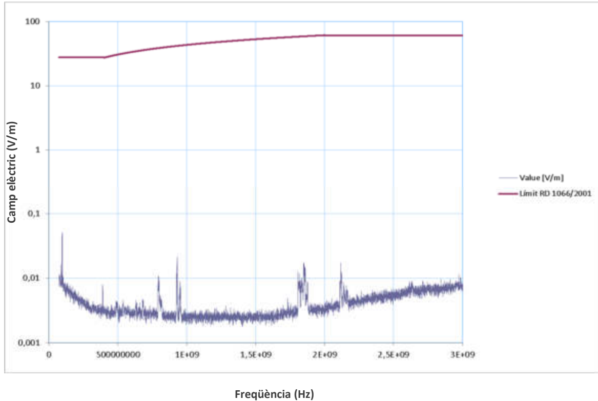
Figura 10. Valors de camp elèctric obtinguts per les freqüències entre 75 MHz i 3 GHz al punt 10.
