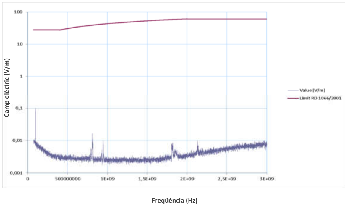
Figura 11. Valors de camp elèctric obtinguts per les freqüències entre 75 MHz i 3 GHz al punt 11.
