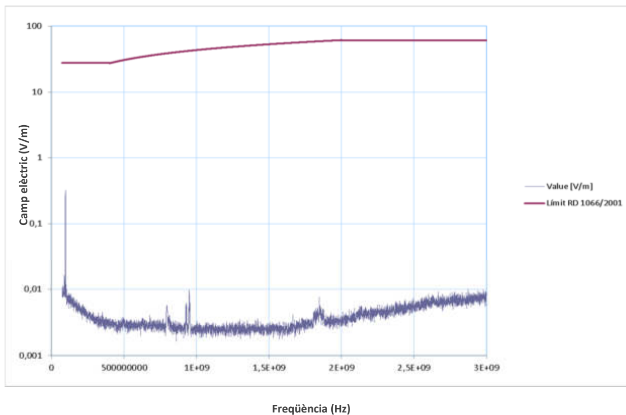
Figura 7. Valors de camp elèctric obtinguts per les freqüències entre 75 MHz i 3 GHz al punt 7.
