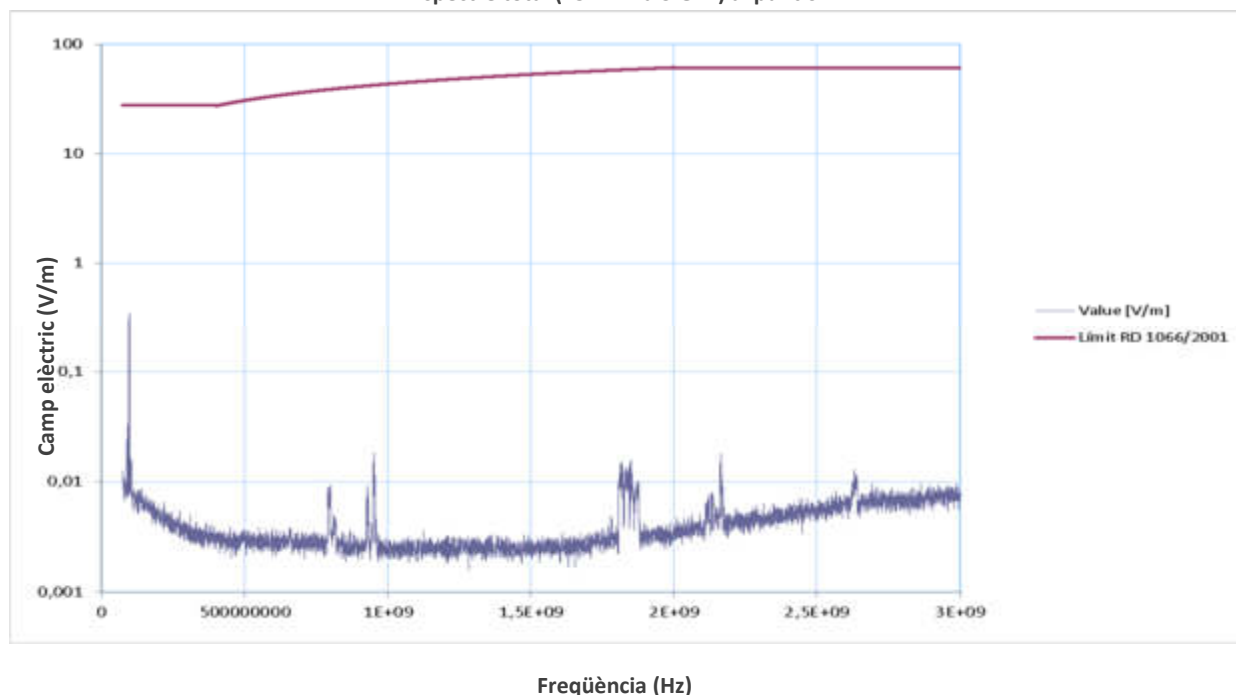
Figura 6. Valors de camp elèctric obtinguts per les freqüències entre 75 MHz i 3 GHz al punt 6.
