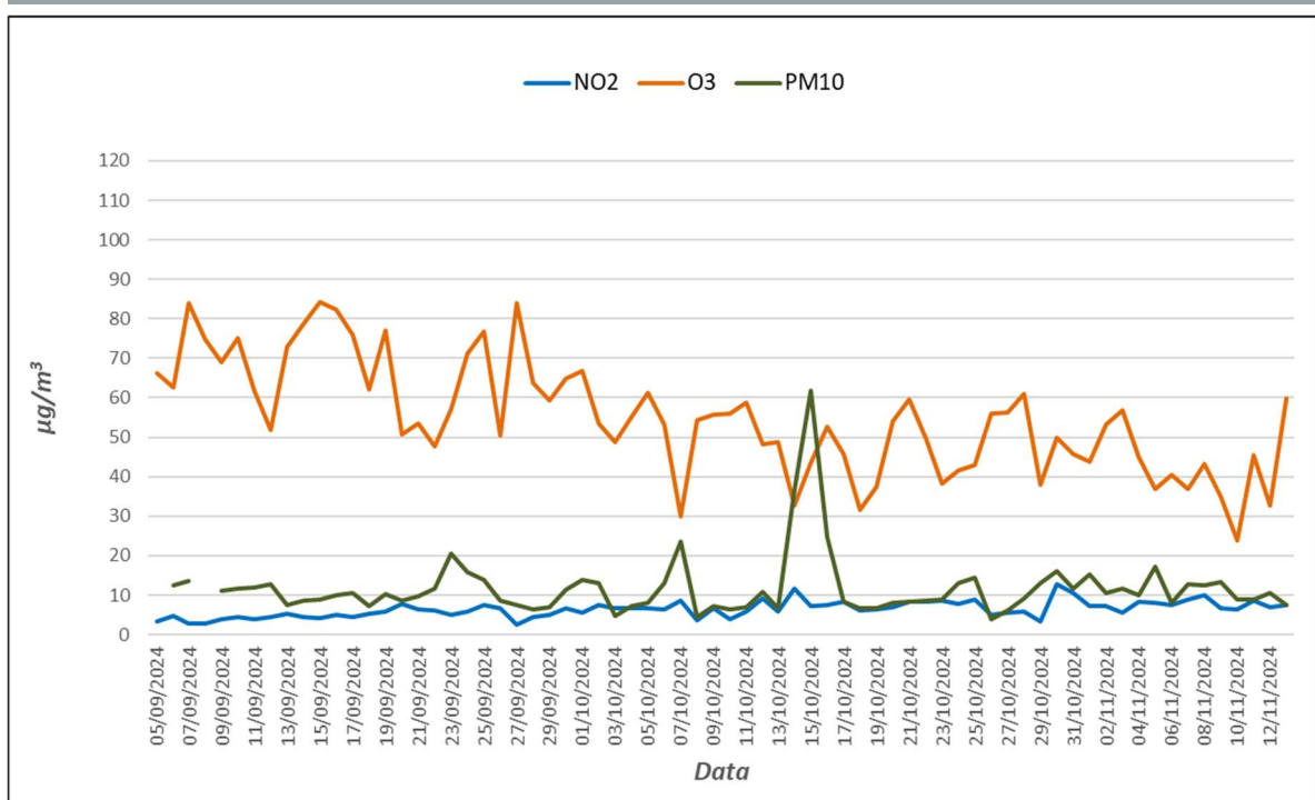
Figura 10. Evolució diària dels contaminants.
