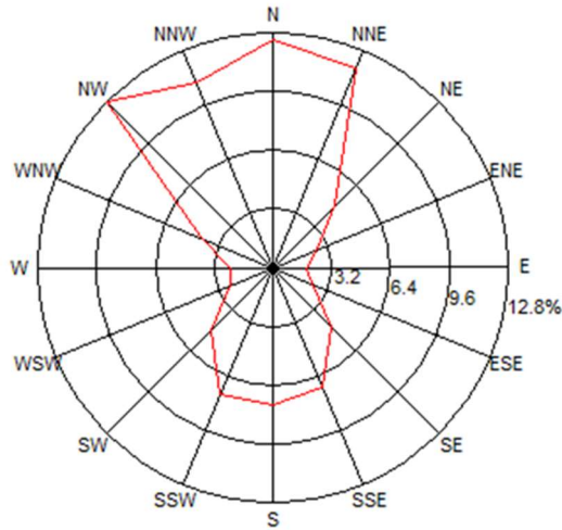
Figura 4. Gràfiques de vent a Avià.
