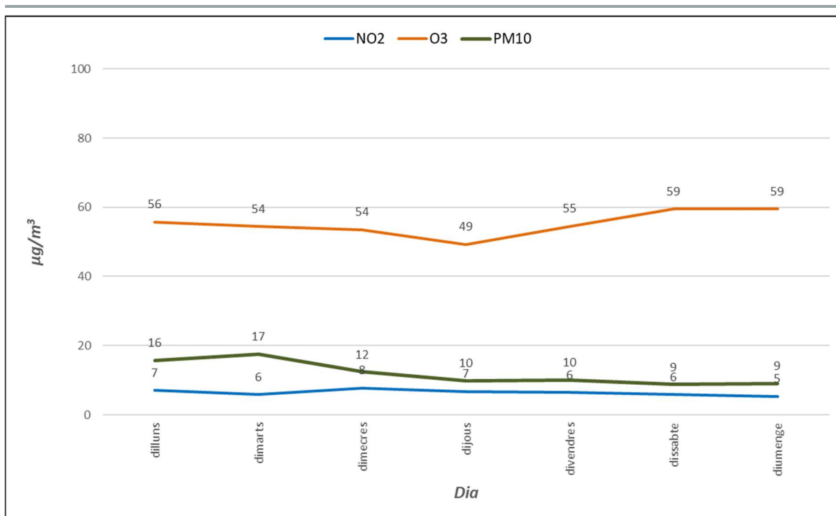
Figura 12. Evolució dels contaminats en la setmana tipus.
