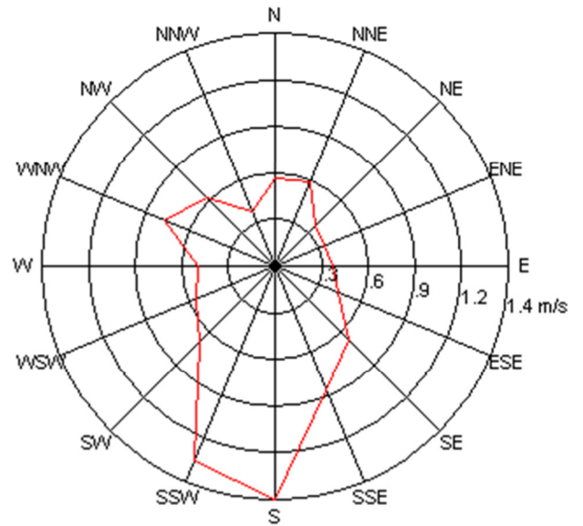
Velocitat del vent - Unitat Mòbil 1 - 06/07/2023 al 12/09/2023
