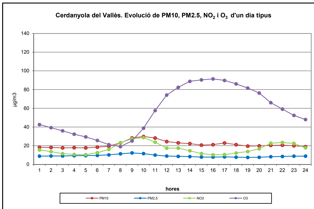
Figura 12. Gràfic del dia tipus dels diferents contaminants
