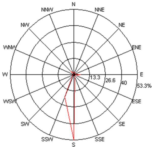
Freqüència del vent - Unitat Mòbil 1 - 06/07/2023 al 12/09/2023
