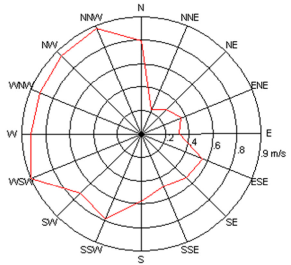
Velocitat del vent - Unitat Mòbil 3 - 22/02/2023 al 01/05/2023
