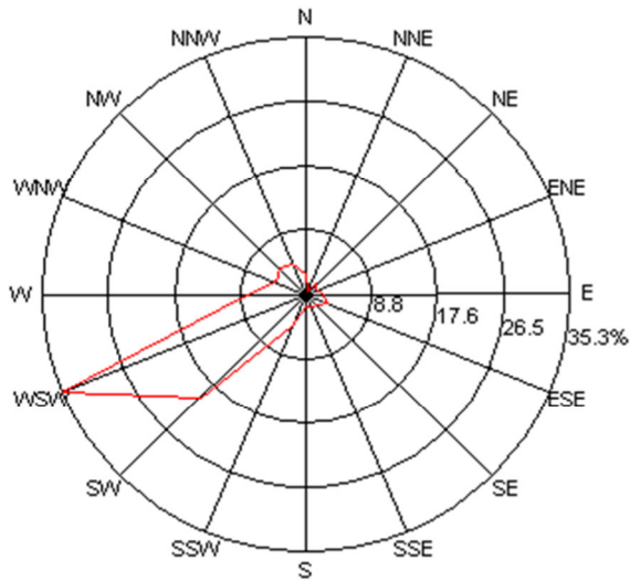
Freqüència del vent - Unitat Mòbil 3 - 22/02/2023 al 01/05/2023
