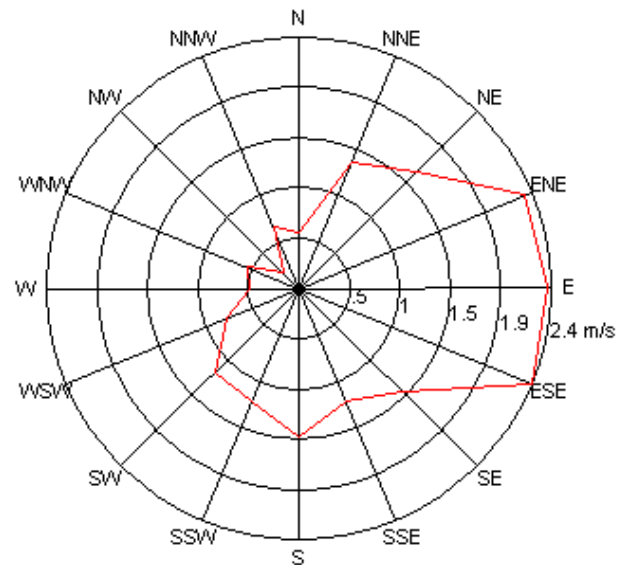
Velocitat del vent - Unitat Mòbil 1 - 14/09/2023 al 20/11/2023
