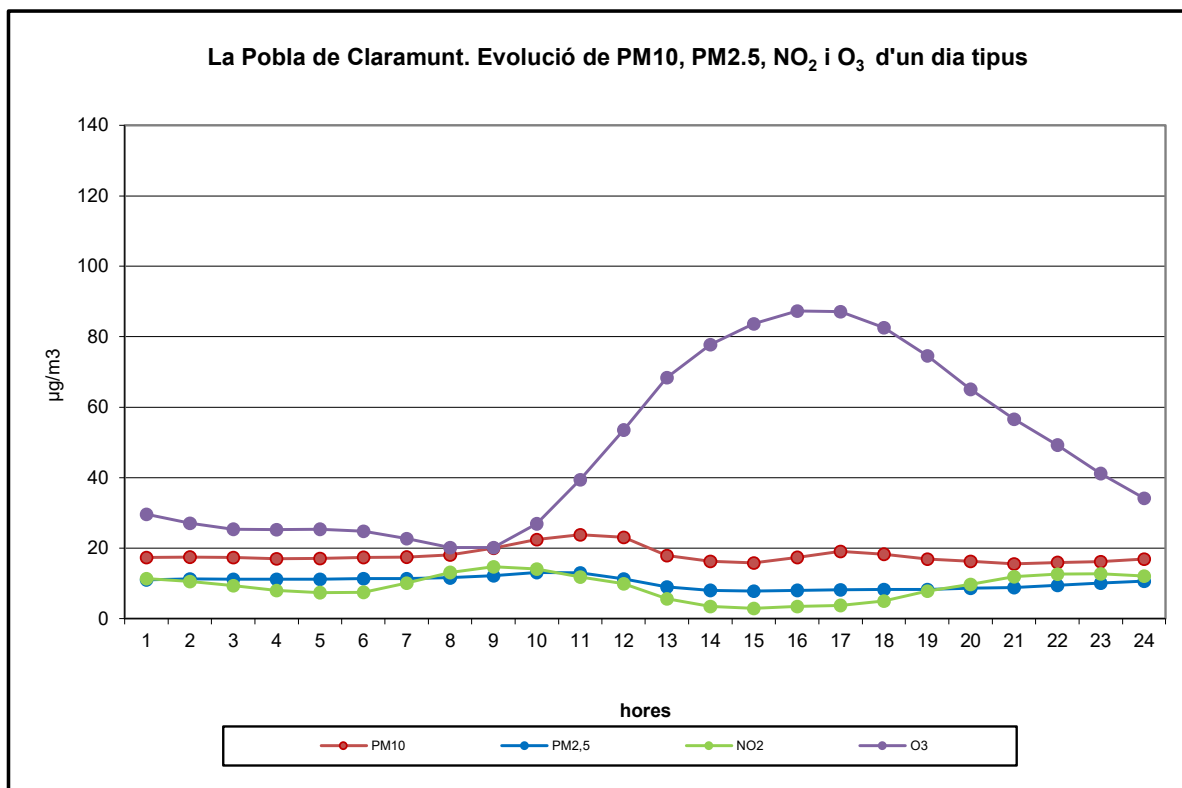
Figura 11. Gràfic del dia tipus dels diferents contaminants
