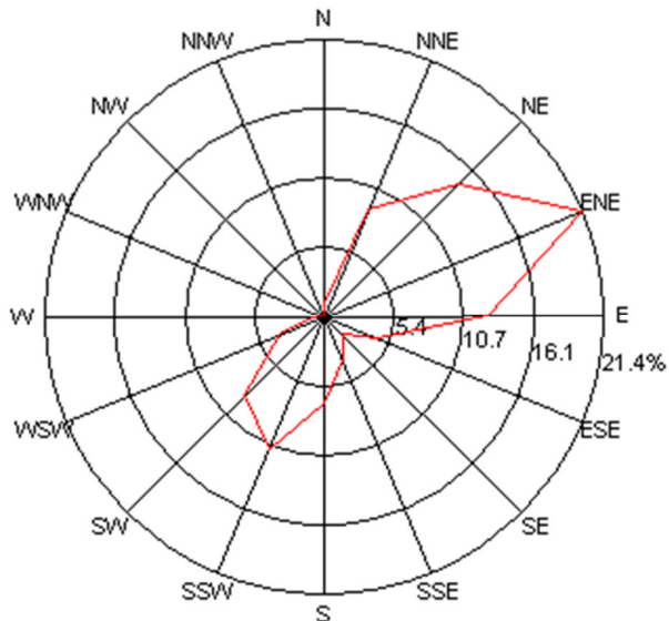
Freqüència del vent - Unitat Mòbil 1 - 14/09/2023 al 20/11/2023
